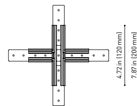
X-JOINT
