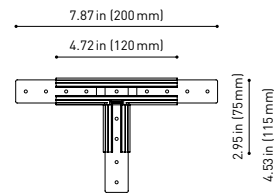
L-JOINT
