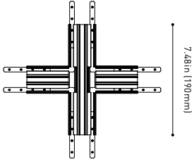
X-JOINT
