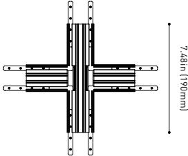
X-JOINT
